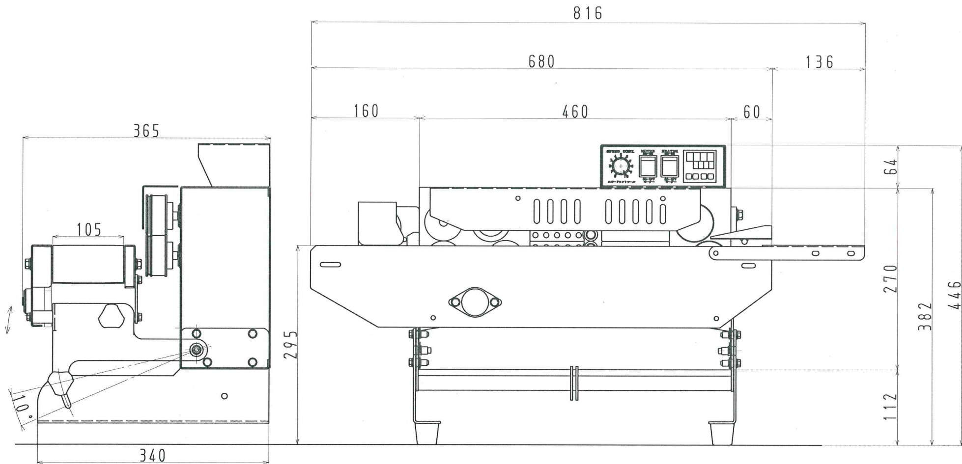
SLE-Cタイプ外形寸法図
